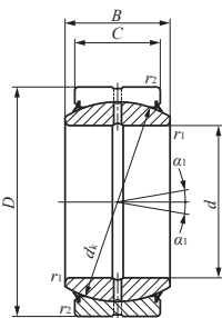
GE...ES-2RS
