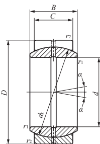
GE...ES
